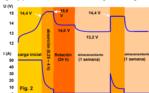
Curvas de carga: hasta la tensión de gaseado (fig.1) y por encima de la tensión de gaseado (fig.2)
